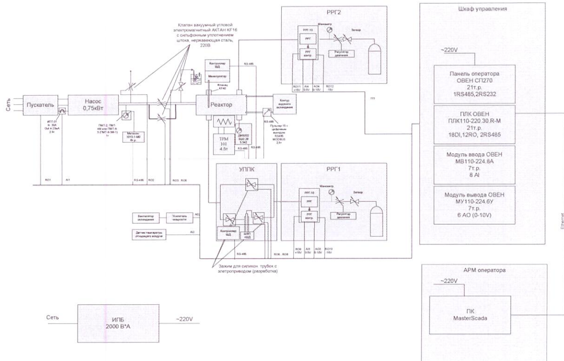
Рисунок 1. Структурная схема
